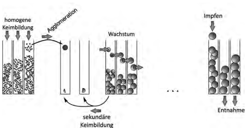
Abb. 1: Populationsbilanz
