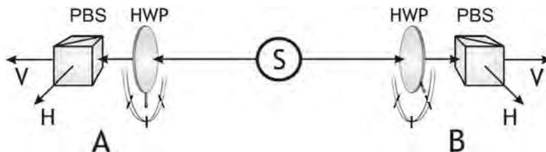
Abbildung 2: Experiment mit Photonenpaaren. Die Quelle S erzeugt Photonenpaare. Eines der Photonen wird zu Messapparat A , das andere Photon zu Messapparat B geschickt. Die Polarisation jedes Photons wird mit einem polarisierenden Strahlteiler (PBS) gemessen. Je nachdem, ob das Photon horizontal oder vertikal polarisiert ist, kommt es im H -Strahl oder V -Strahl heraus und kann dort nachgewiesen werden. Die Messung der Polarisation entlang verschiedener Richtungen erreicht man durch die Halbwellenplatte (HWP). Diese dreht die Polarisation des Photons um einen gewissen Winkel, der von der Orientierung der Halbwellenplatte abhängt. Die Messung der Polarisation mit feststehendem PBS und gedrehter HWP ist genau so, als wenn man die Messung mit einem gedrehten PBS gemacht hätte. Man kann damit die Polarisation entlang einer beliebigen Richtung messen.
